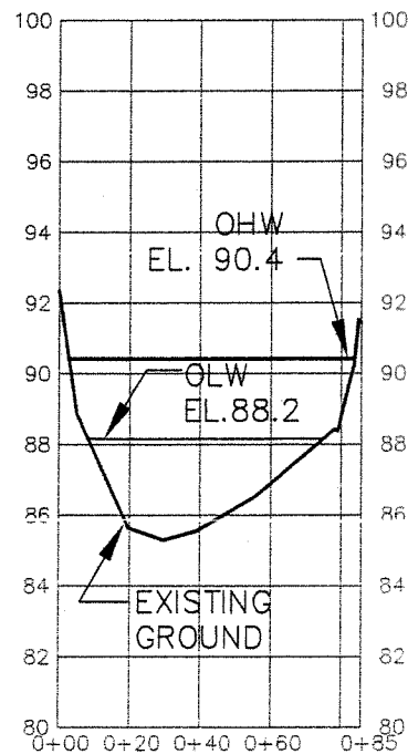
SECTION B-B' STA 1643
