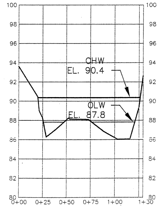
SECTION C-C' STA 1975
