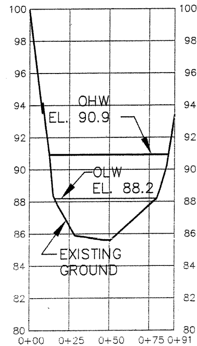
SECTION A-A' STA 1562
