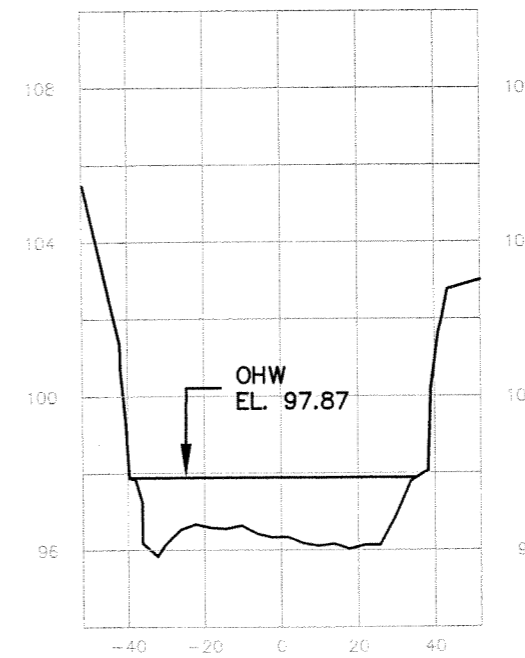
SECTION 6 STA 11+50
