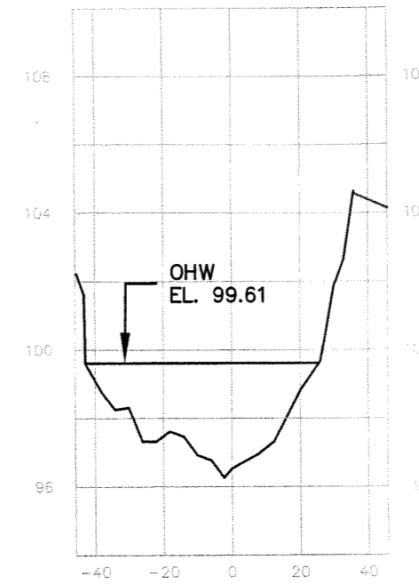
SECTION 3 STA 3+98
