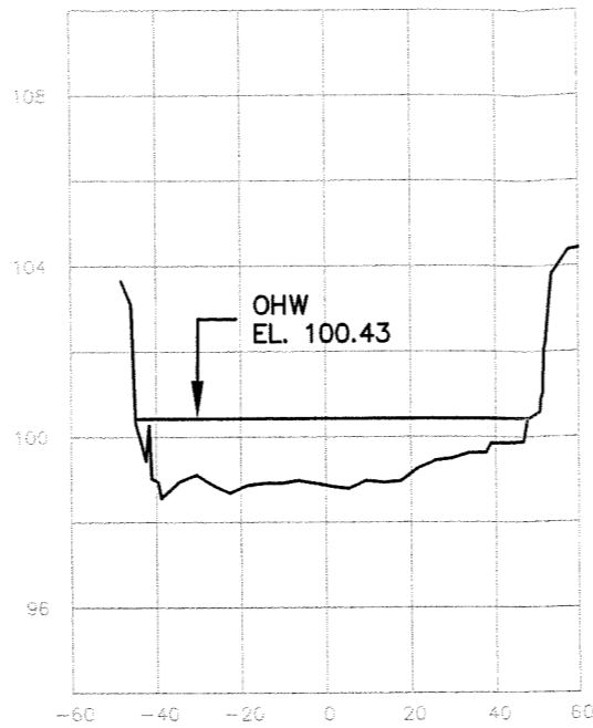
SECTION 2 STA 2+44
