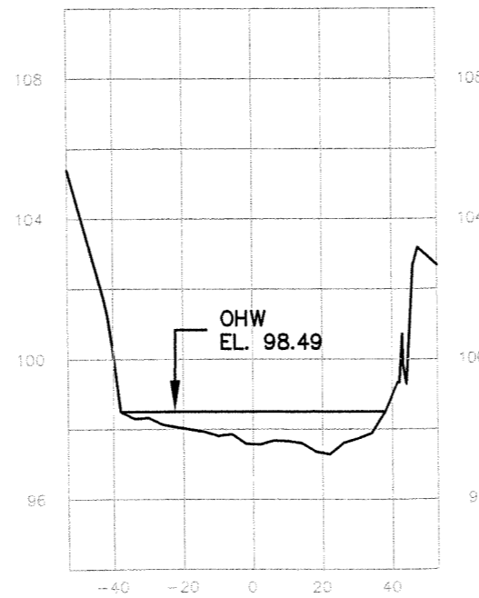
SECTION 5 STA 10+14
