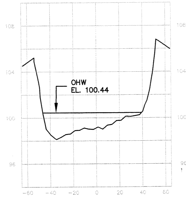
SECTION 1 STA 1+17
