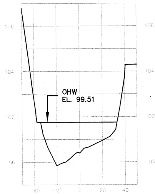
SECTION 4 STA 5+88
